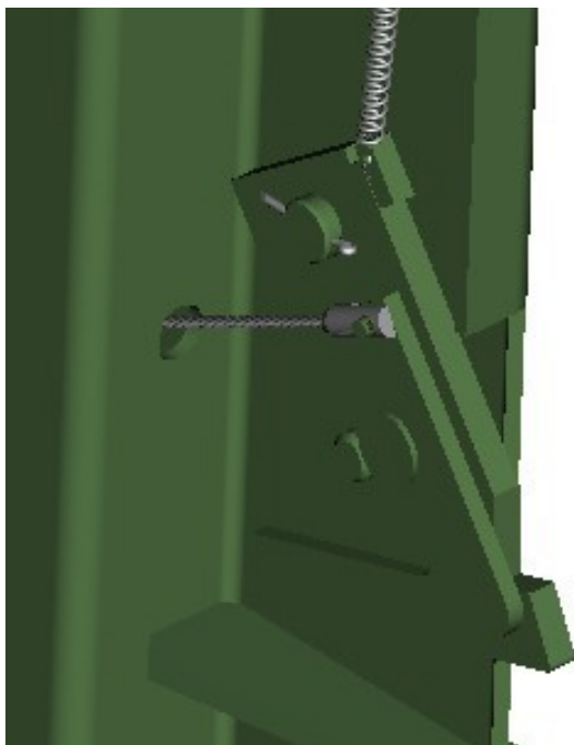
Предохранительная пластина в положении зацепления
